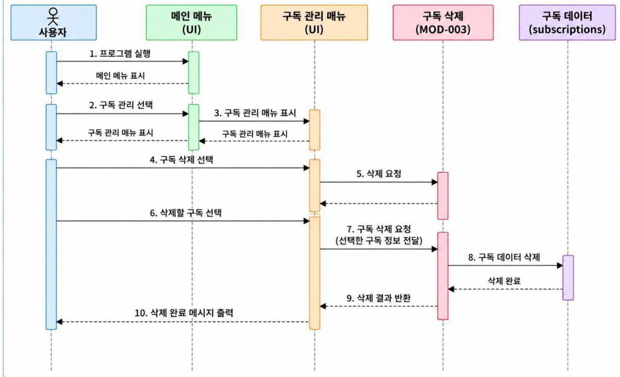
구독삭제 시퀀스 다이어그램
