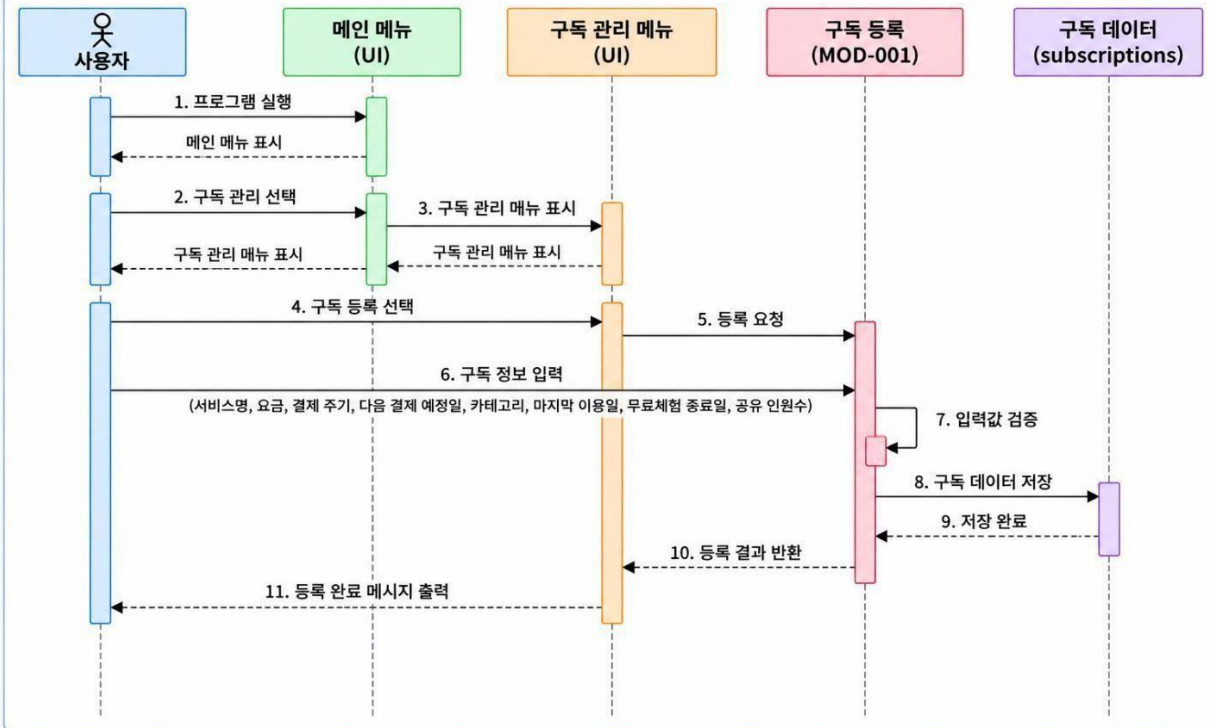
구독등록 시퀀스 다이어그램
